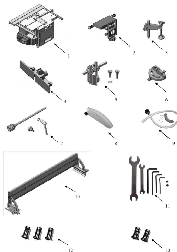
Obr. 7: Jednotlivé díly stroje při dodání
