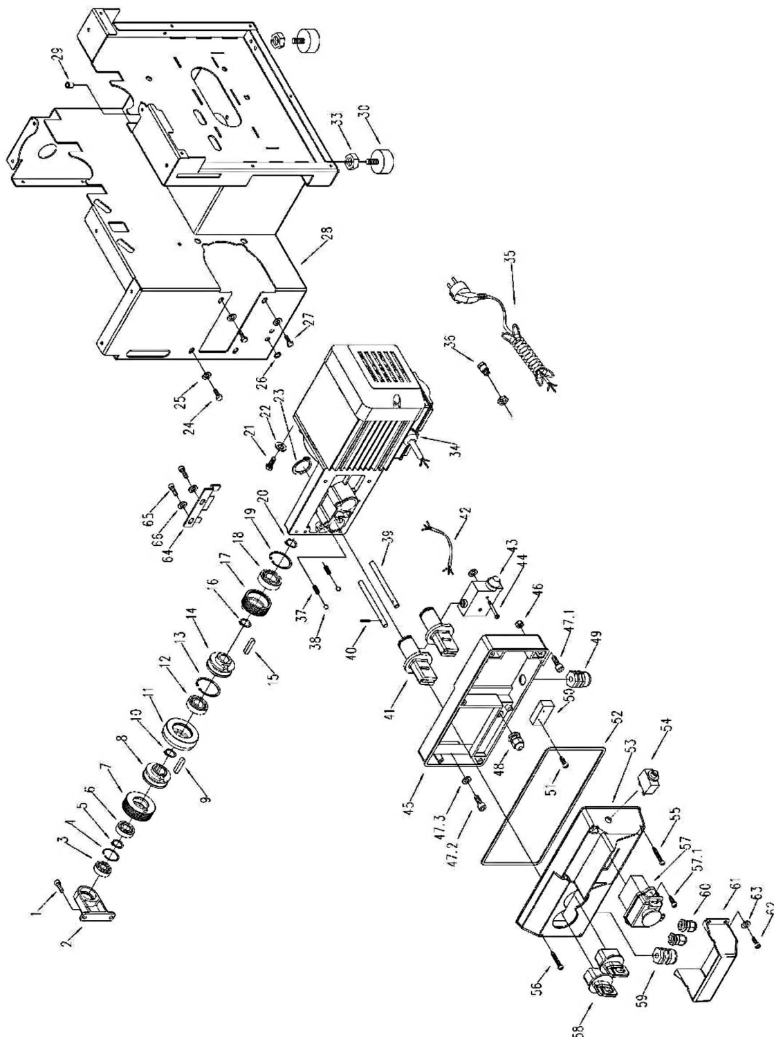
Obr. 49: Rozpadové schéma 1
